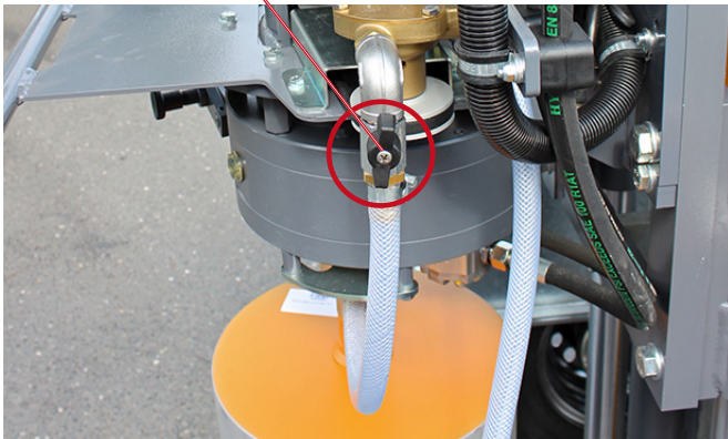
Wasserabsperrhahn geöffnet
