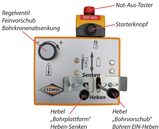
Bedienpult
