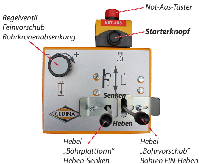
Bedienpult
