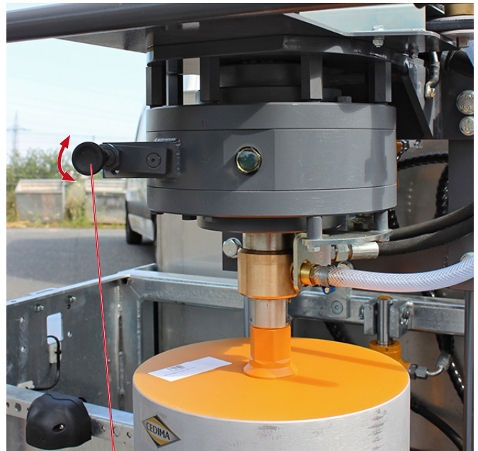
Getriebestellhebel mit Rastbolzen zum einstellen der Drehzahl
